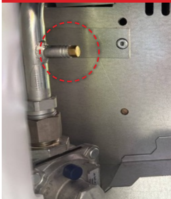
CAPUCHON DE GAZ DU PORT D'ESSAI INCLUS
